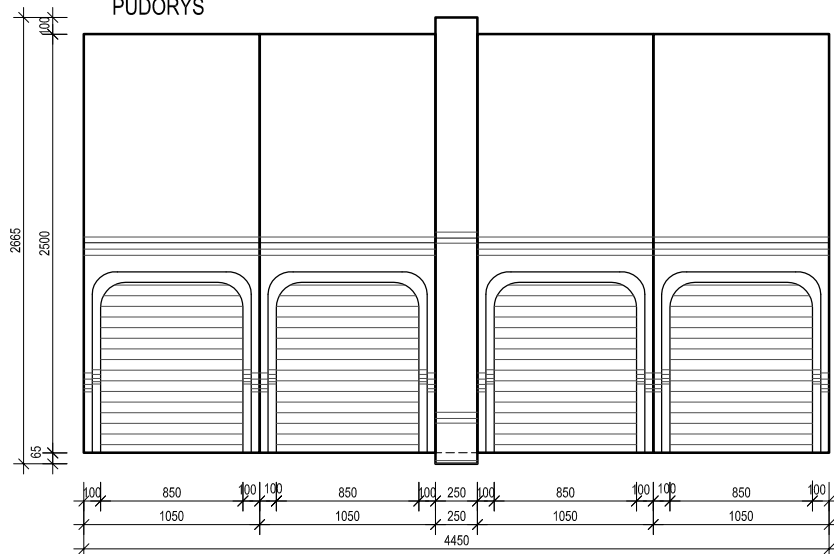
PŮDORYS
